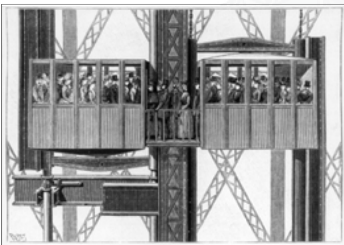
Ascenseur Edoux pour aller du 2 e au 3 e étage de la Tour de 300 m – Disposition des cages au plancher intermédiaire pour le transbordement des voyageurs à 240 m d'altitude
