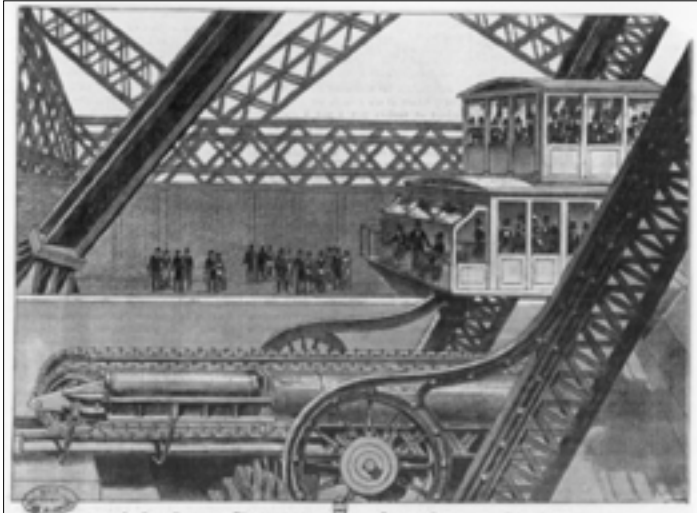
Mécanisme des ascenseurs Roux et Combaluzier
